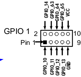
GPIO1 Header
